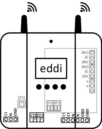
Figuur 9 Elektrische aansluitingen eddi met relais en sensorbord (vereenvoudigde weergave)
