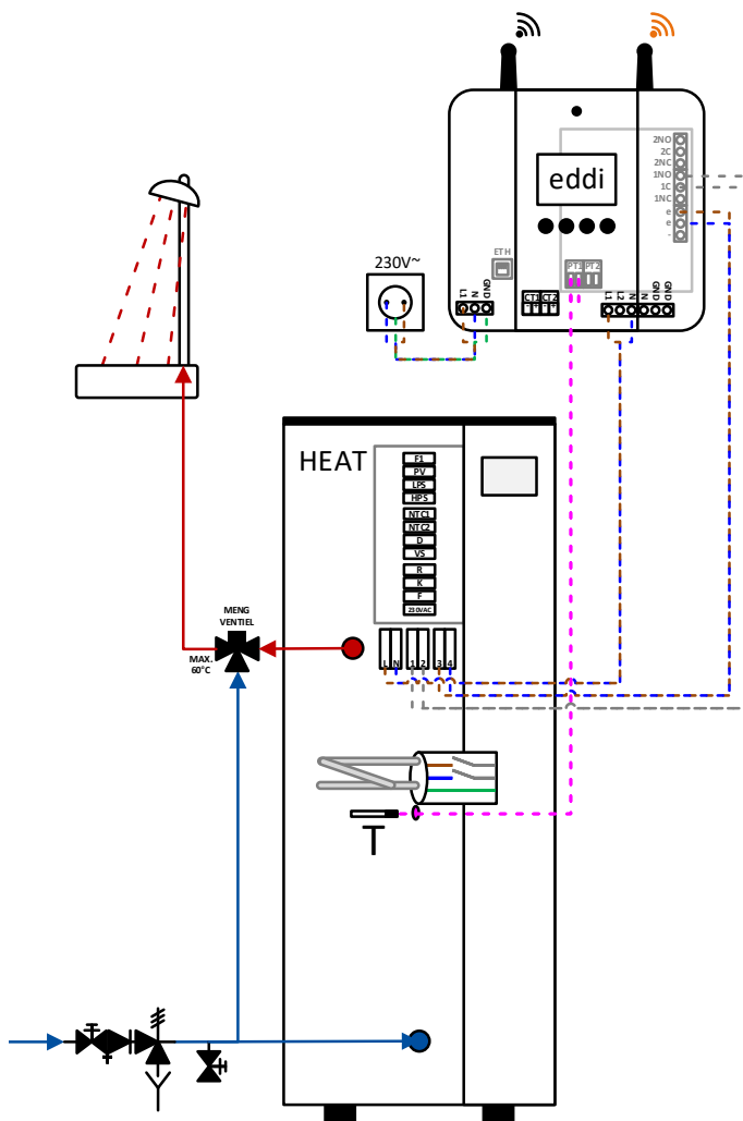
Figuur 6 Sunsmart Heat – Elektrisch aansluitschema
