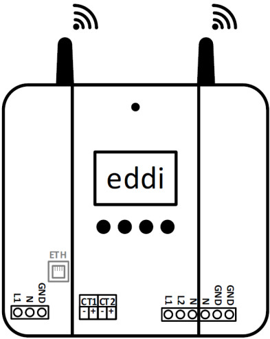
Figuur 8 Elektrische aansluitingen eddi (vereenvoudigde weergave)
